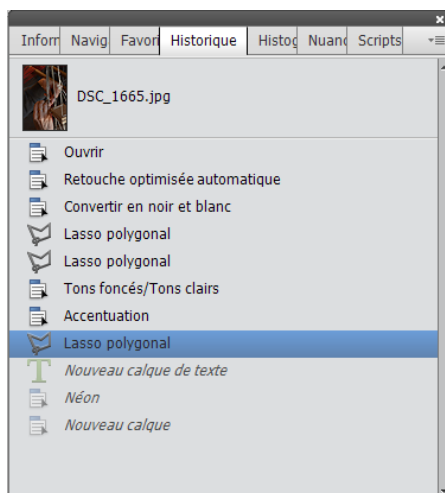
Fenêtre d'historique
